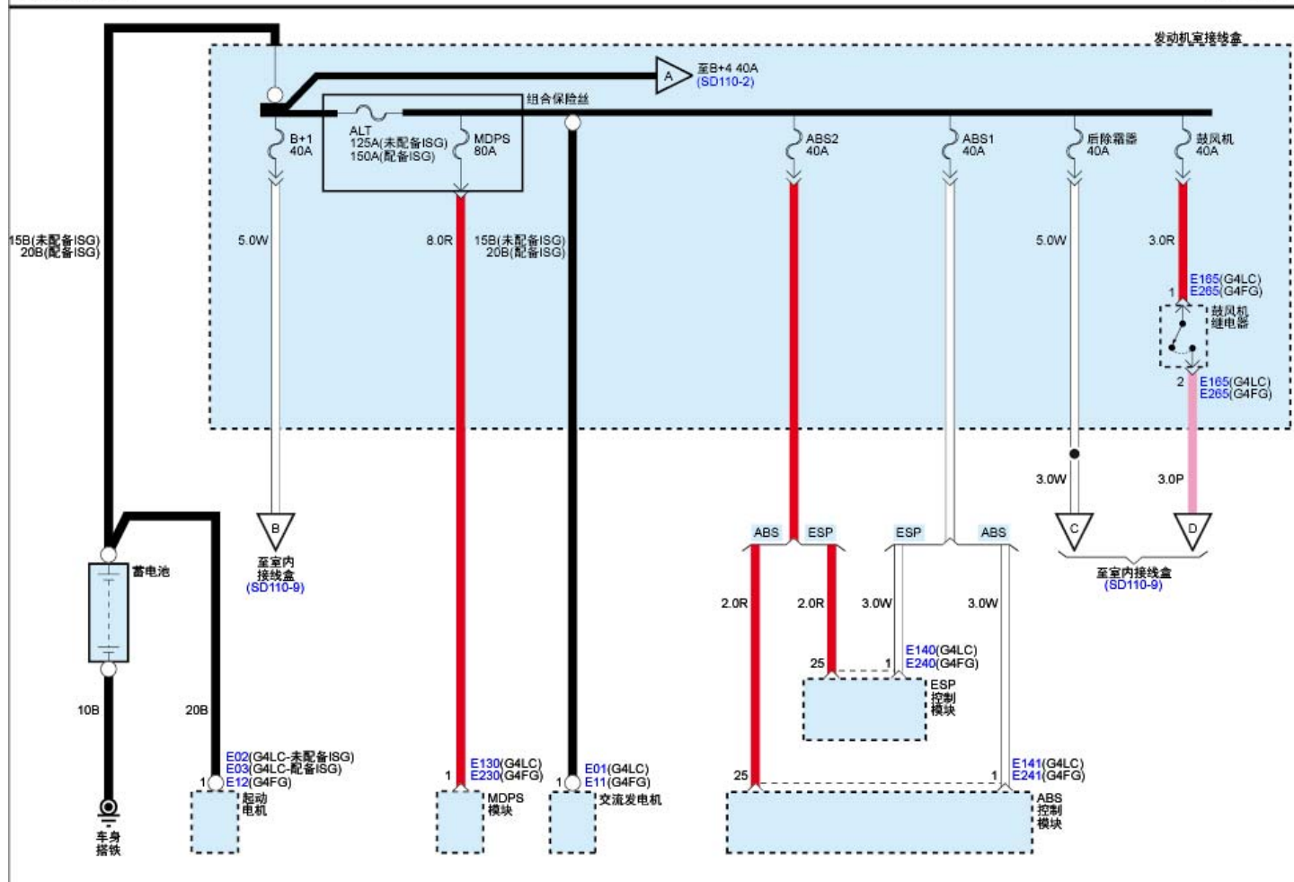
电源分布(1)
